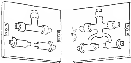
FIG. 517. MATCH PLATE.
